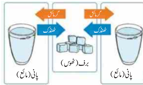
شکل 1.2 رجعی تعامل
