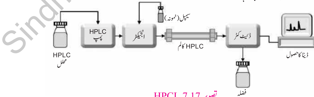
تصویر 7.17 HPLC
