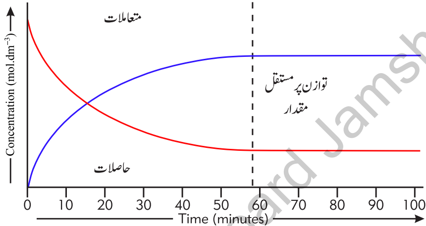
شکل 1.4 متحرک توازن
