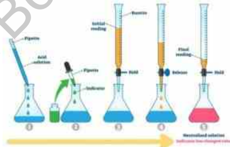
تصویر 7.12 ٹائٹریشن
